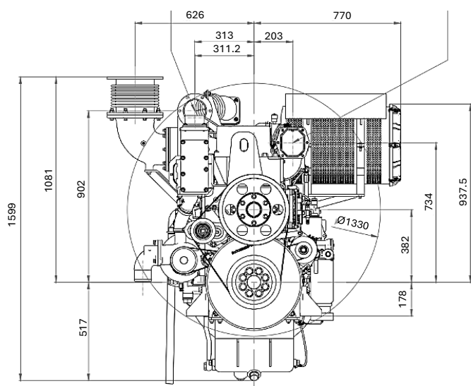
FRONT VIEW- FAN
